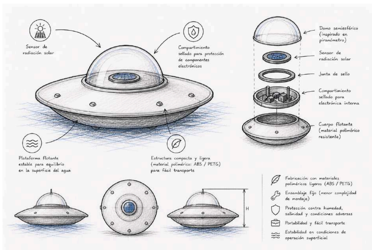
Figura 10: solución Mecánica 1
