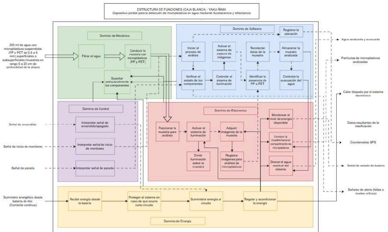
Figura 6: Estructura de funciones de YAKU-ÑAWI.
