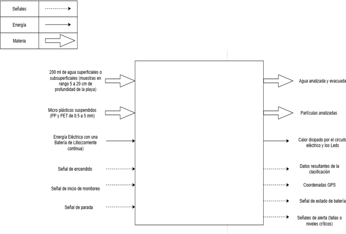
Figura 4: Caja Negra de YAKU-ÑAWI.
