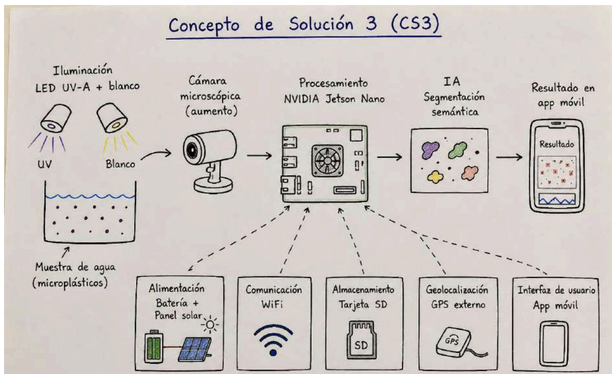
Figura 9: Concepto de solución 3.
