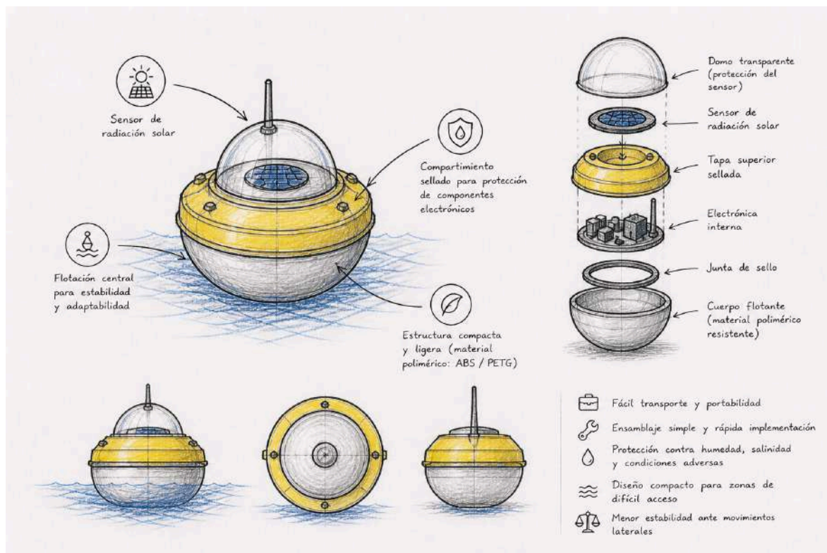
Figura 12: solución Mecánica 3
