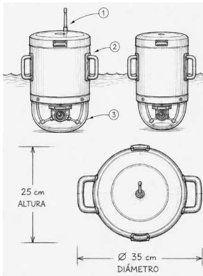
Figura 15.1: Vista perspectiva general del Boceto 3.
