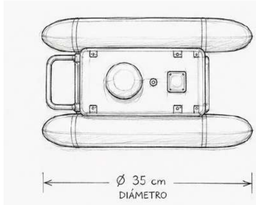
Figura 14.3: Vista frontal del Boceto 2
